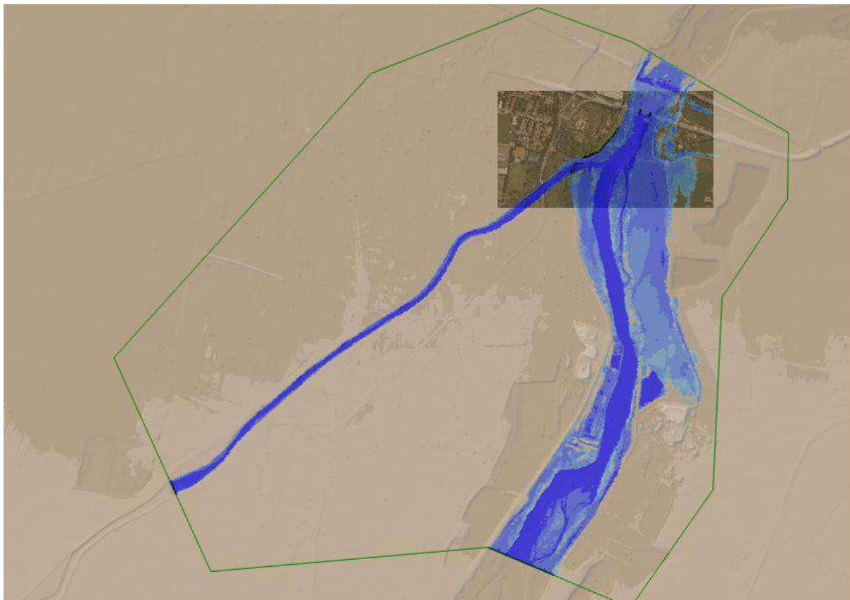
Figura 28 - Vista del modello idraulico bidimensionale - aree allagabili per TR200 di entrambi i corpi idrici - SDP
