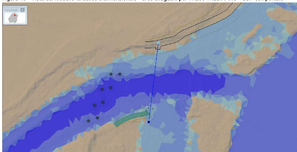
Figura 41 - Dettaglio delle aree allagabili e della sezione in corrispondenza della passerella in progetto – SDP portale
