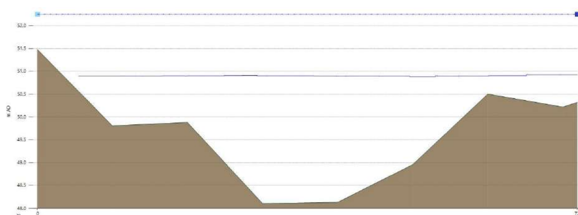
Figura 17 - Vista della sezione e del tirante idrico in corrispondenza della sezione della passerella in progetto
