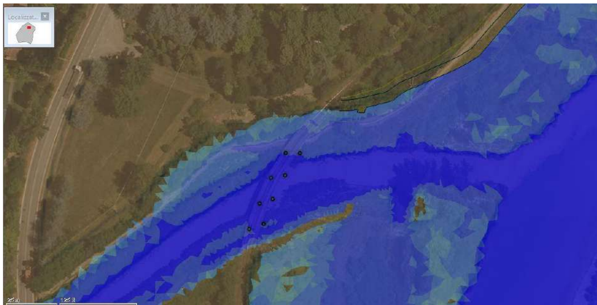
Figura 29 - Dettaglio delle aree allagabili e della sezione in corrispondenza della passerella in progetto
