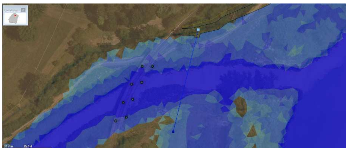
Figura 16 - Dettaglio delle aree allagabili e della sezione in corrispondenza della passerella in progetto
