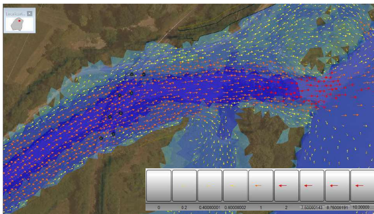
Figura 35 - Vista dei vettori velocità in corrispondenza dei tiranti massimi nell'area della passerella
