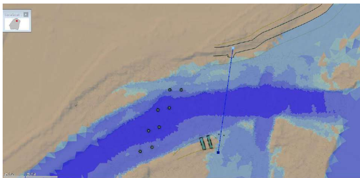
Figura 37 - Dettaglio delle aree allagabili e della sezione in corrispondenza della passerella in progetto (SDP con portale e scatolari)
