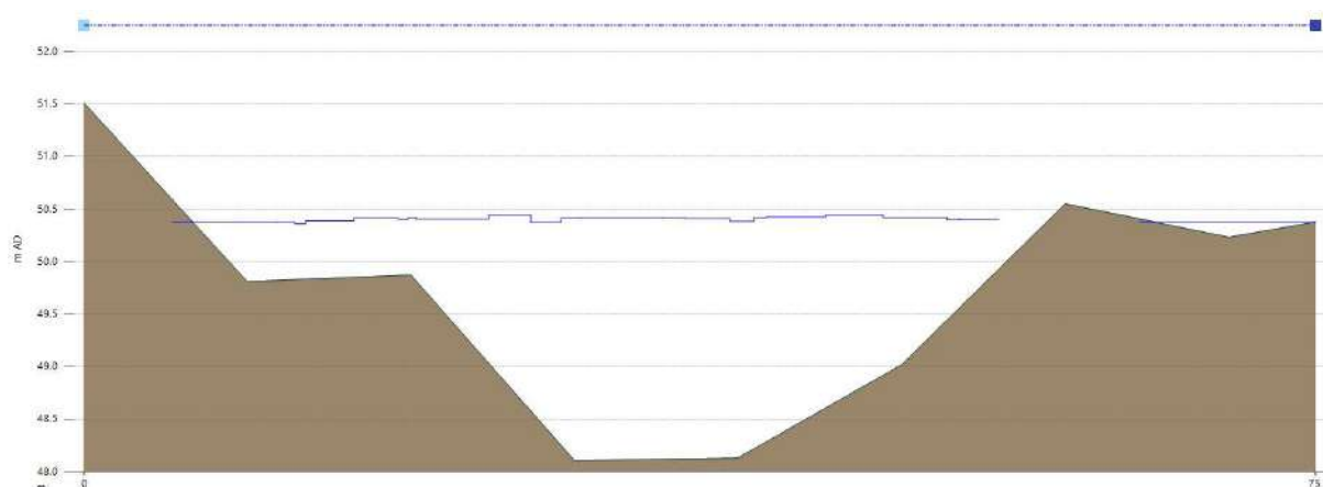
Figura 22 - Vista della sezione e del tirante idrico in corrispondenza della sezione della passerella in progetto
