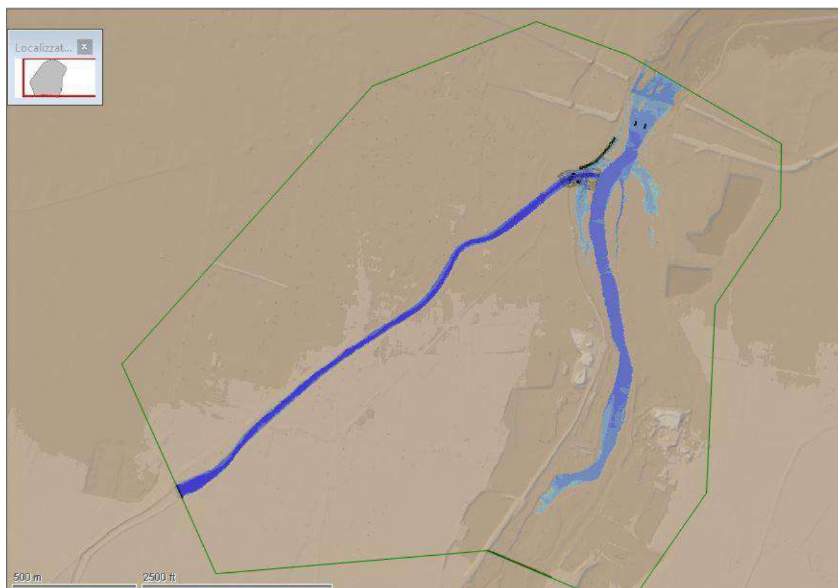
Figura 36 - Vista del modello idraulico bidimensionale - aree allagabili per TR200 TRESINARO – SDP portale + scatolari
