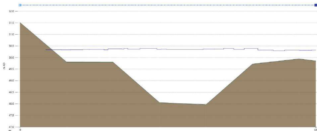
Figura 42 - Vista della sezione e del tirante idrico in corrispondenza della sezione della passerella in progetto – SDP portale
