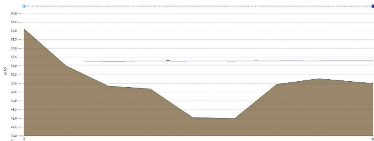
Figura 25 - Vista della sezione e del tirante idrico in corrispondenza della sezione della passerella in progetto
