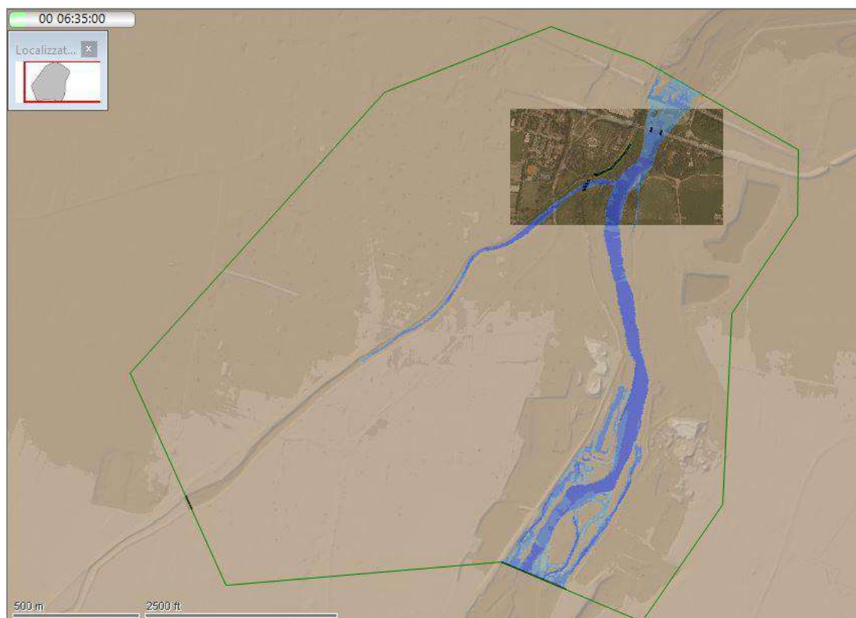
Figura 19 – Estratto della modellazione del Fiume Secchia all'istante 6 ore 35 minuti
