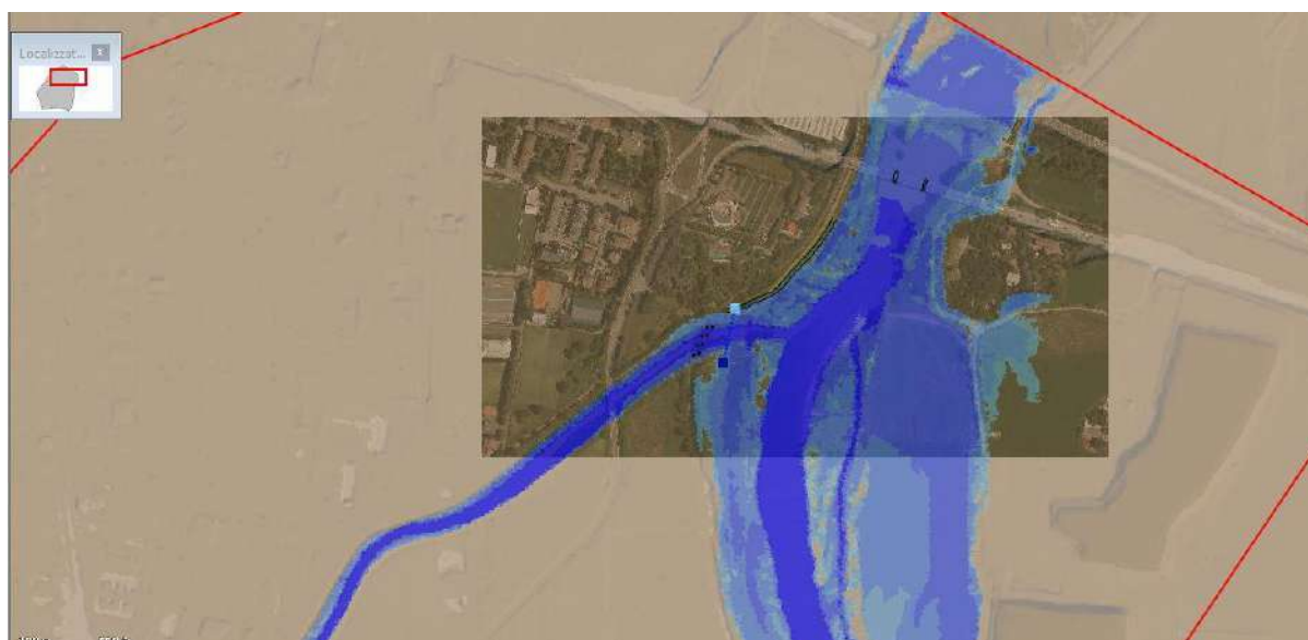
Figura 15 - Vista del modello idraulico bidimensionale - aree allagabili per TR200 del Fiume Secchia
