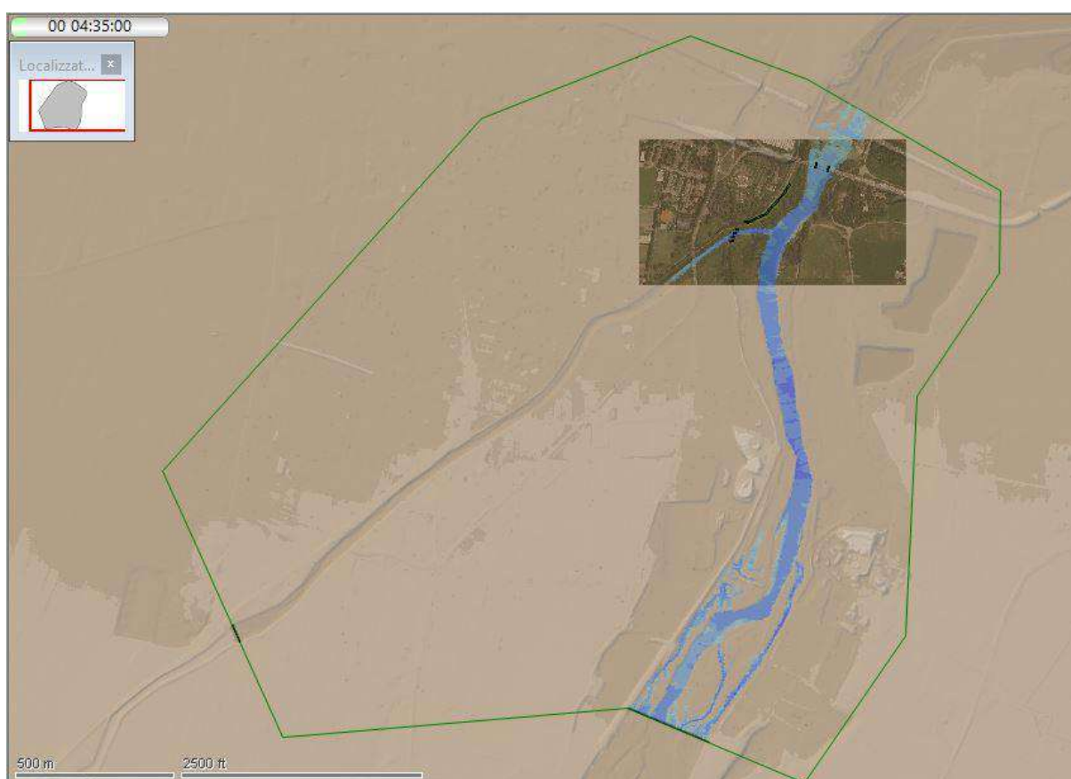
Figura 18 – Estratto della modellazione del fiume Secchia dopo 4 ore e 35 minuti di simulazione (idrogramma)
