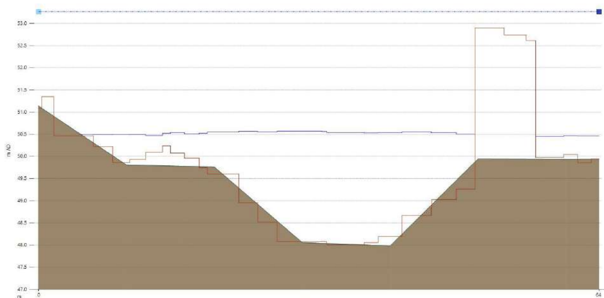
Figura 34 - Vista della sezione e del tirante idrico in corrispondenza della sezione della passerella in progetto
