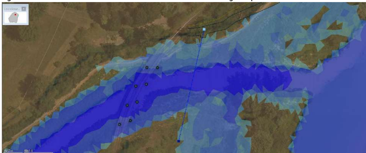
Figura 21 - Dettaglio delle aree allagabili e della sezione in corrispondenza della passerella in progetto
