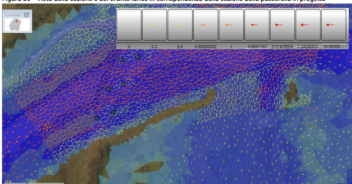
Figura 31 - Vista dei vettori velocità in corrispondenza dei tiranti massimi nell'area della passerella
