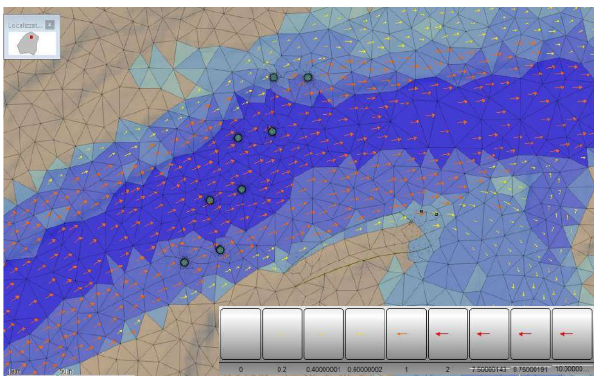
Figura 43 - Vista dei vettori velocità in corrispondenza dei tiranti massimi nell'area della passerella – SDP portale
