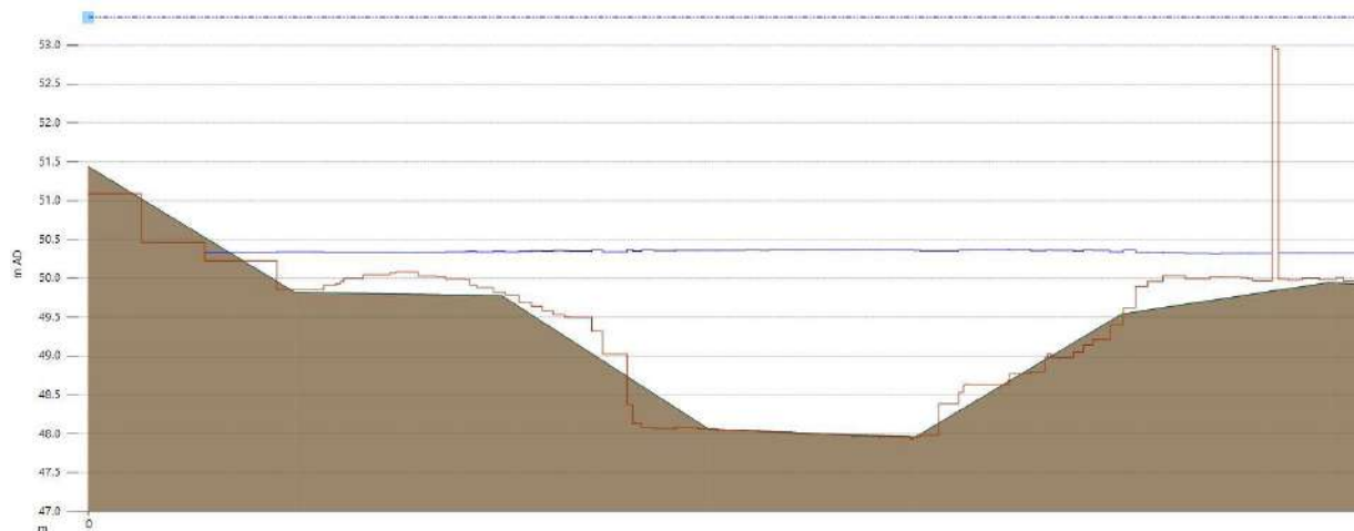
Figura 38 - Vista della sezione e del tirante idrico in corrispondenza della sezione della passerella in progetto (SDP con portale e scatolari)
