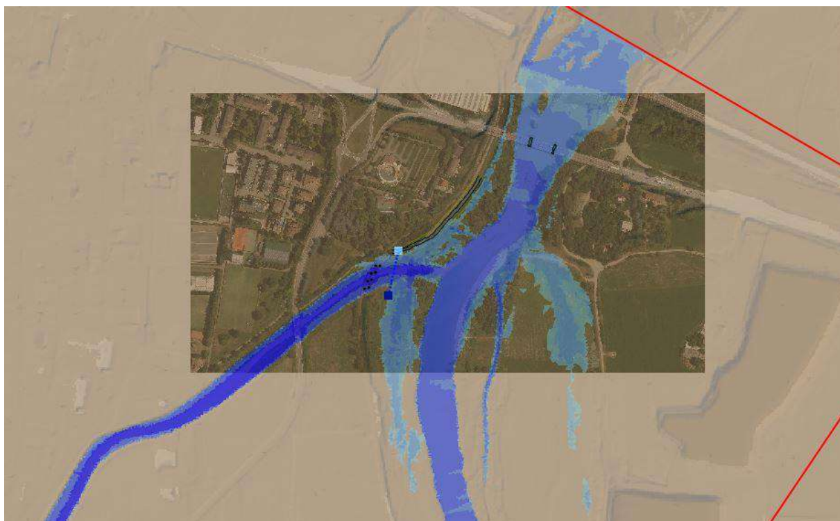
Figura 20 - Vista del modello idraulico bidimensionale - aree allagabili per TR200 del Torrente Tresinaro
