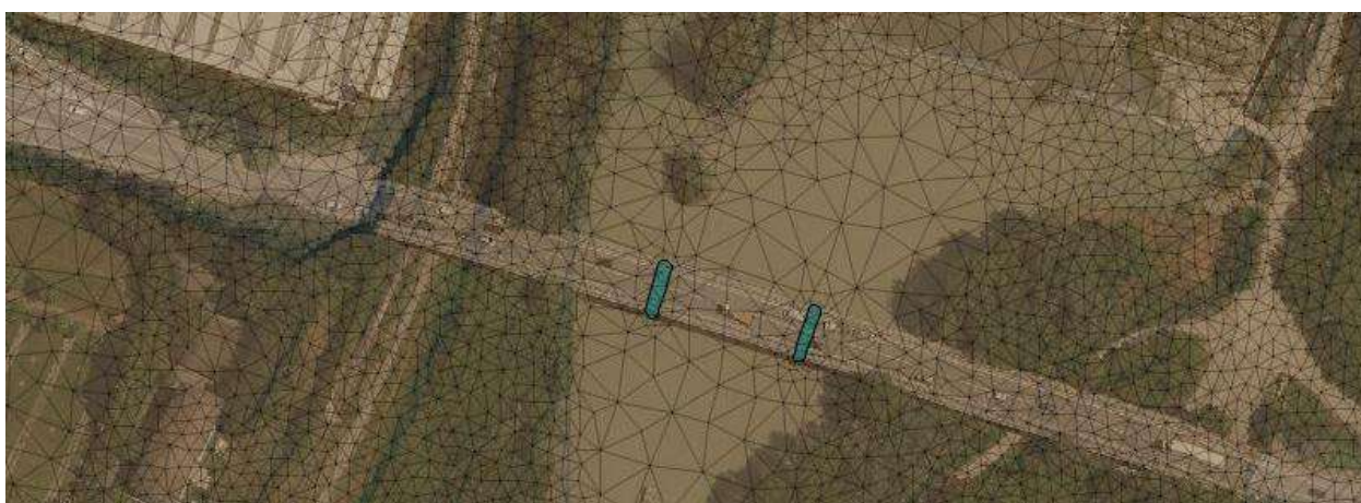
Figura 13 - Estratto del modello (maglia) con indicazione del viadotto della Via Emilia
