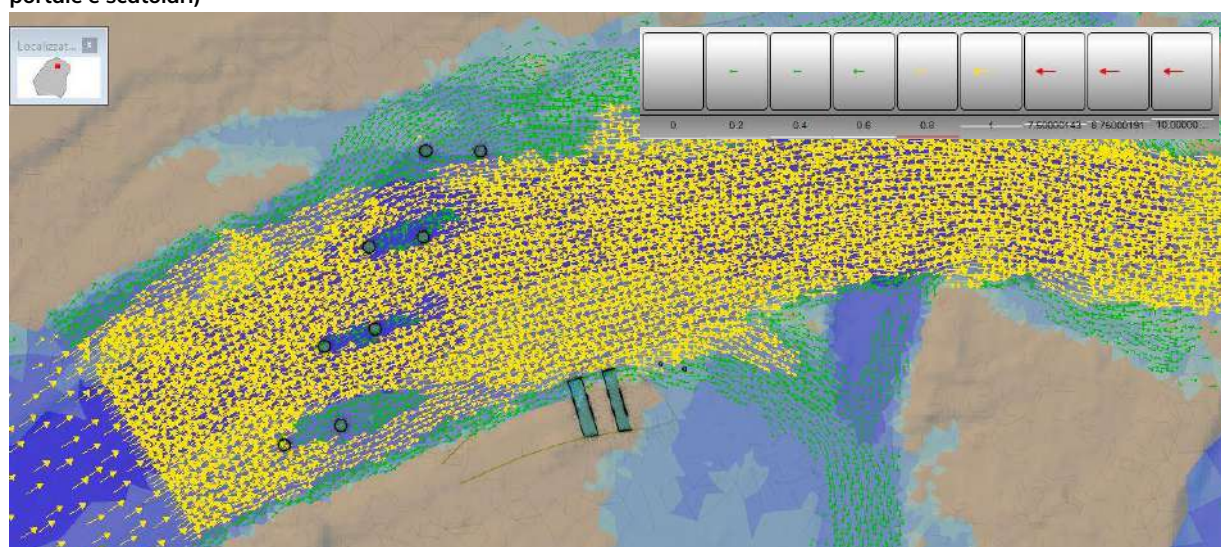
Figura 39 - Vista dei vettori velocità in corrispondenza dei tiranti massimi nell'area della passerella (SDP con portale e scatolari)
