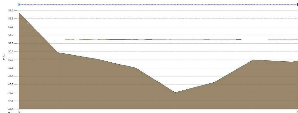
Figura 30 - Vista della sezione e del tirante idrico in corrispondenza della sezione della passerella in progetto
