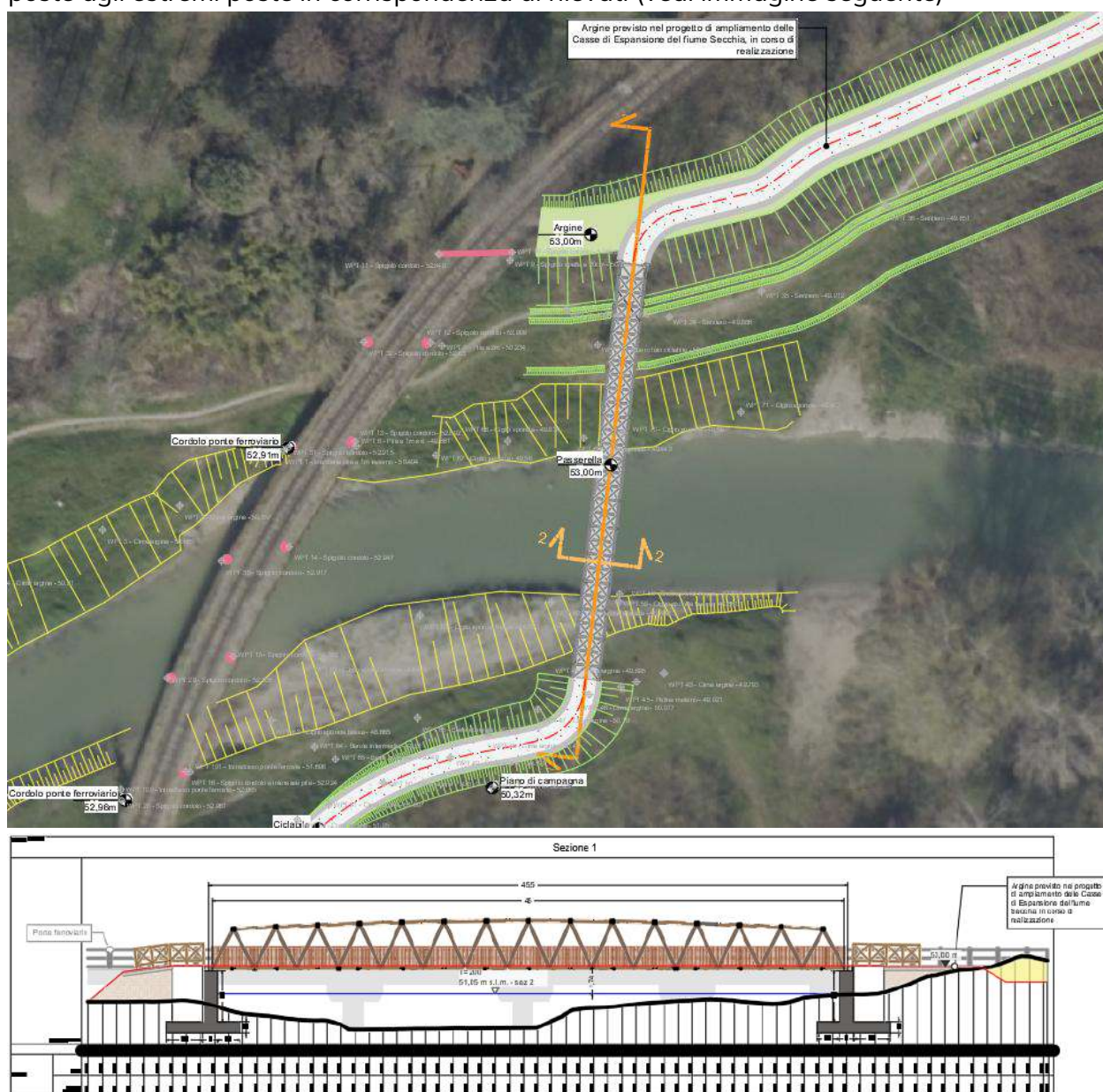
Figura 5 – Sopra: planimetria di progetto; Sotto: Sezione della passerella in progetto - vista da valle (destra idraulica a sinistra)
