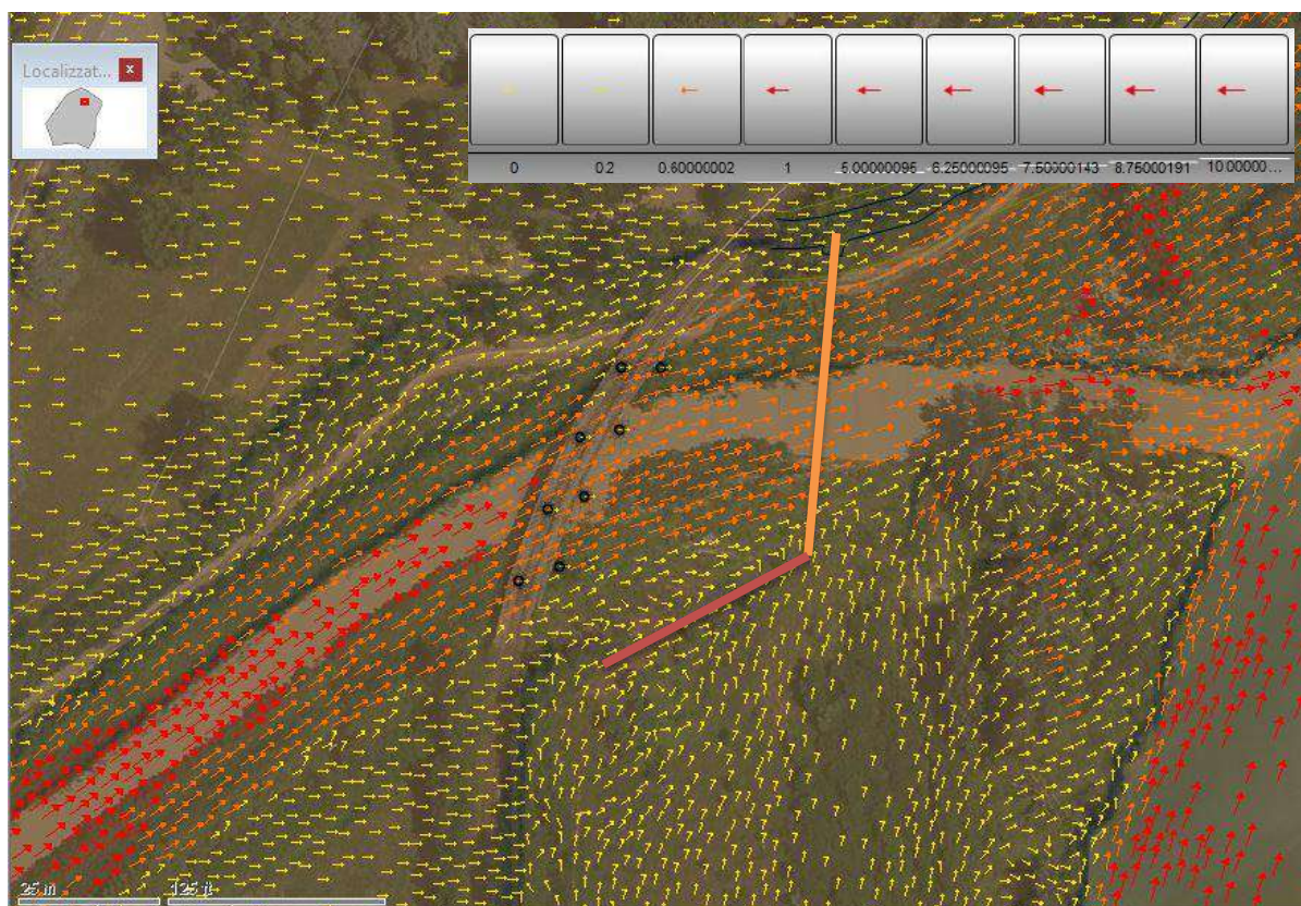
Figura 26 - Estratto del modello idraulico riportante i vettori velocità per lo scenario SDF.3 (linea arancione: posizione passerella in progetto; linea rossa: posizione del rilevato di progetto)
