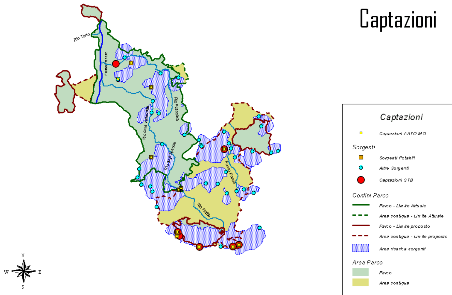
Figura 8 - Captazioni AATO MO e Servizio Tecnico Bacini Enza, Panaro e Secchia di Modena
