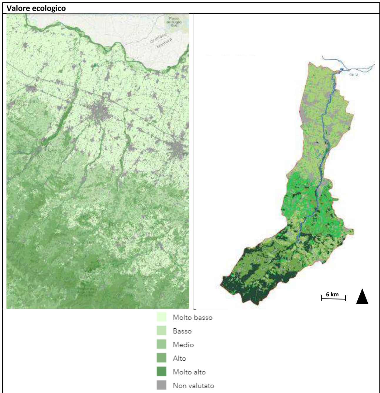
Figura 66 – Valore ecologico del territorio interessato dalla valle dell'Enza (fonte: Carta della Natura)
