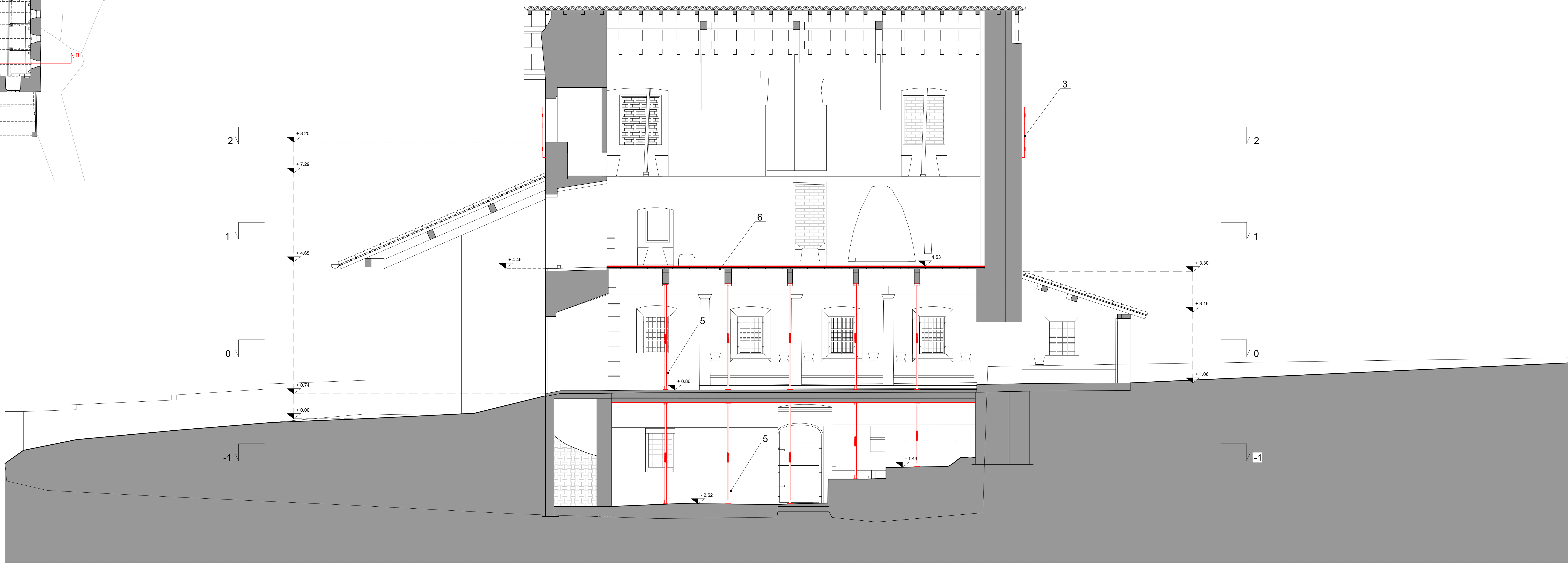
Sezione A-A' - Scala 1:50
