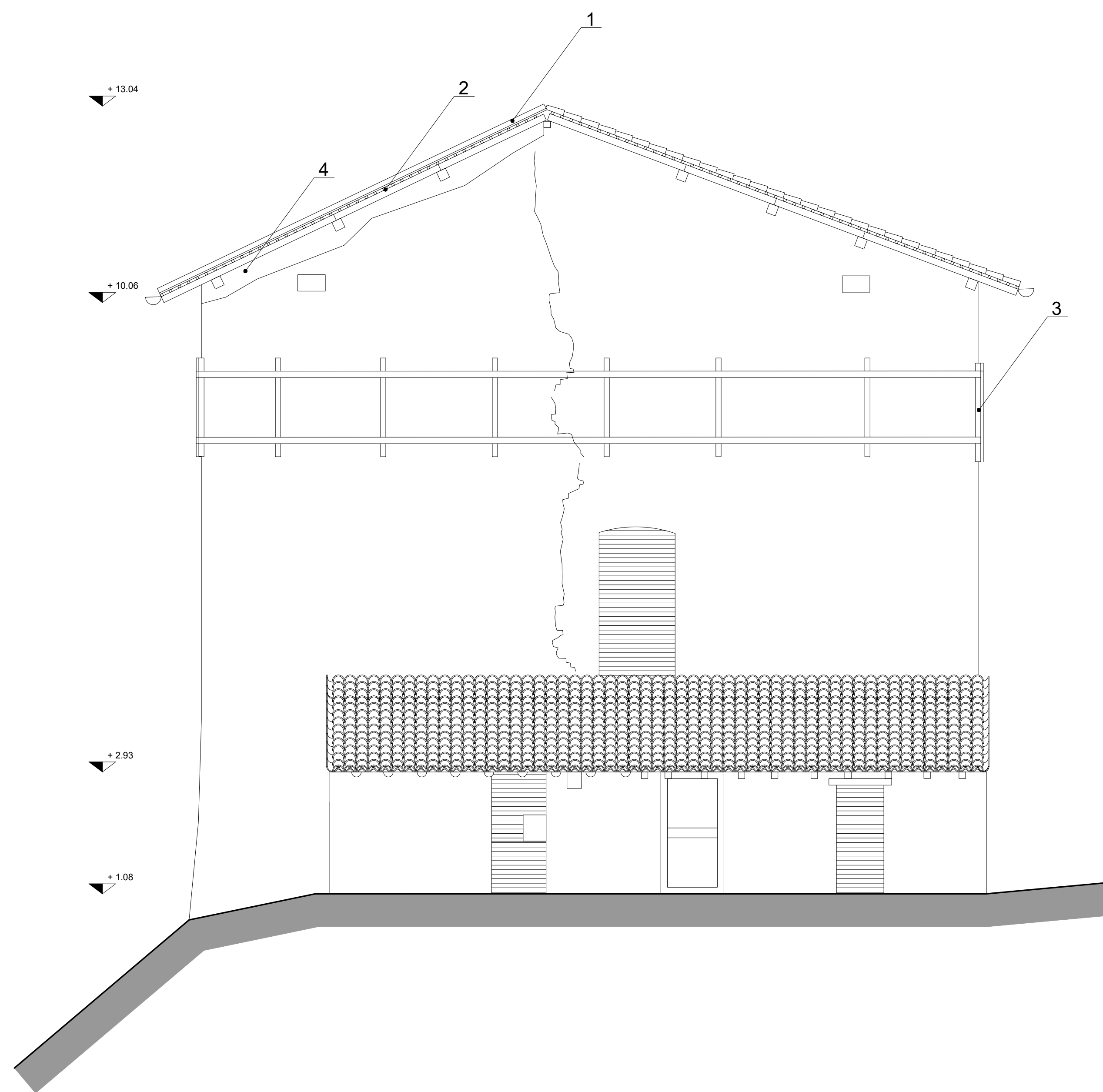
Prospetto Ovest - Scala 1:50
