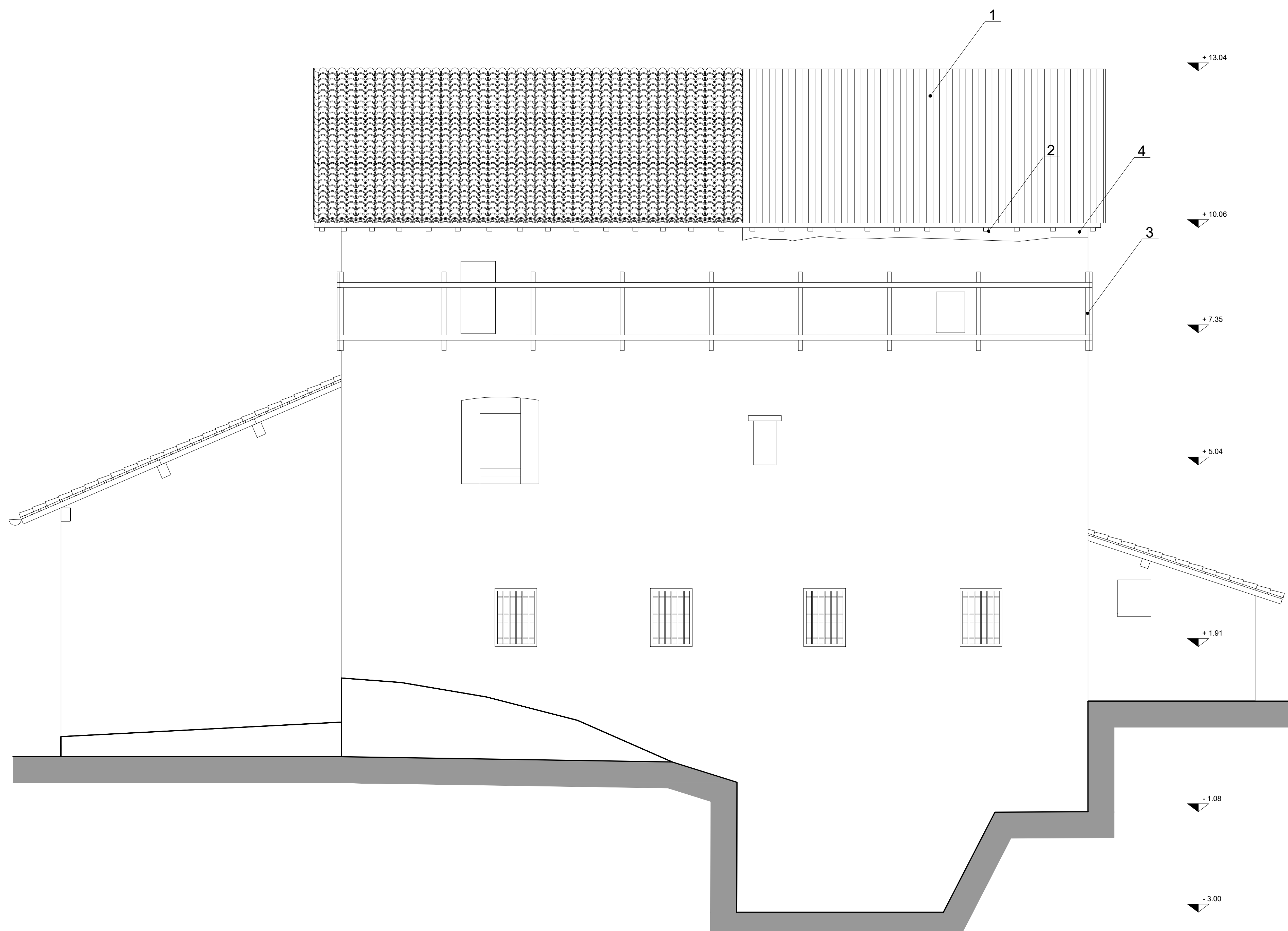
Prospetto Nord - Scala 1:50
