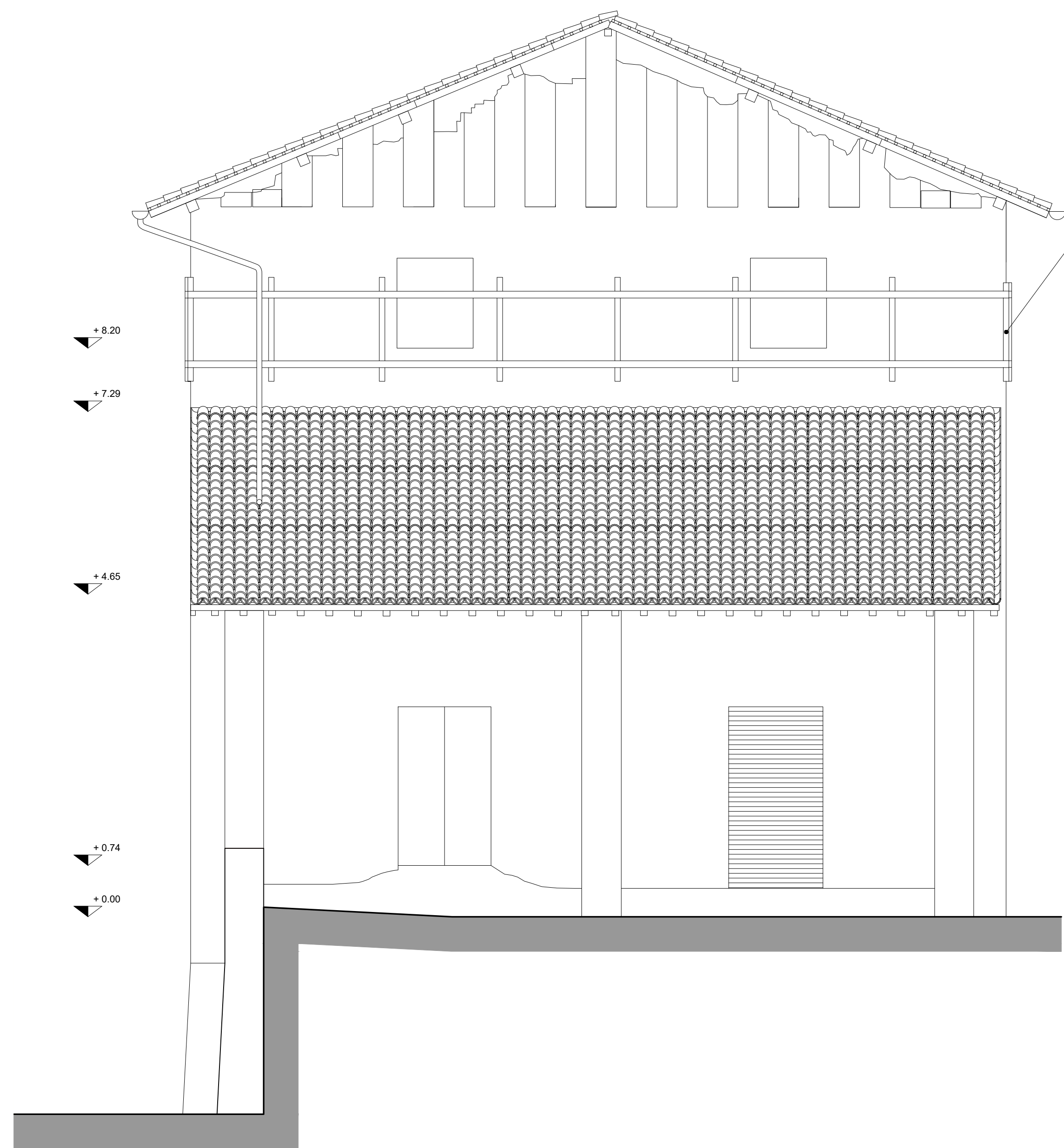
Prospetto Est - Scala 1:50
