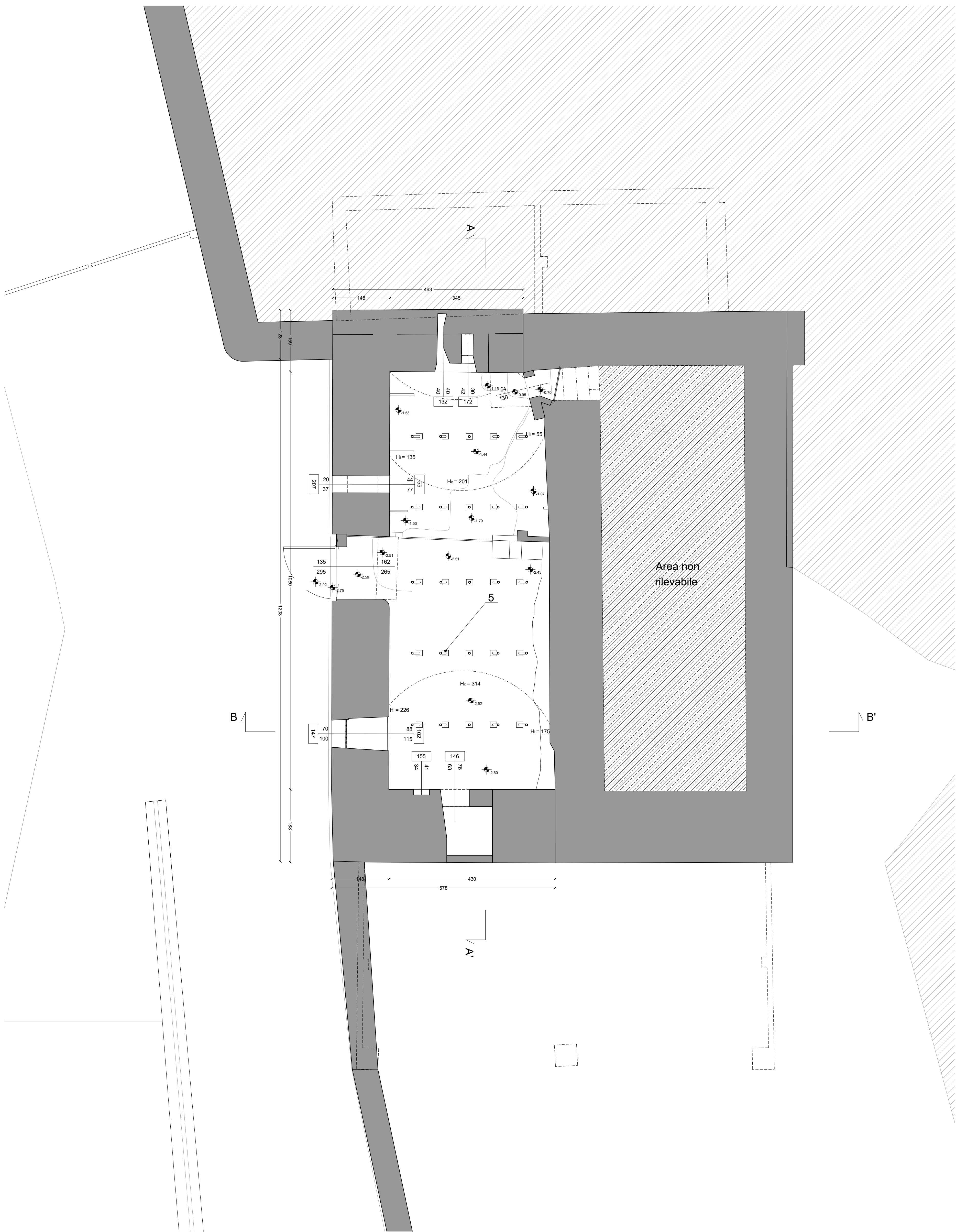
Stato di Progetto - Pianta Livello -1 - 1:50
