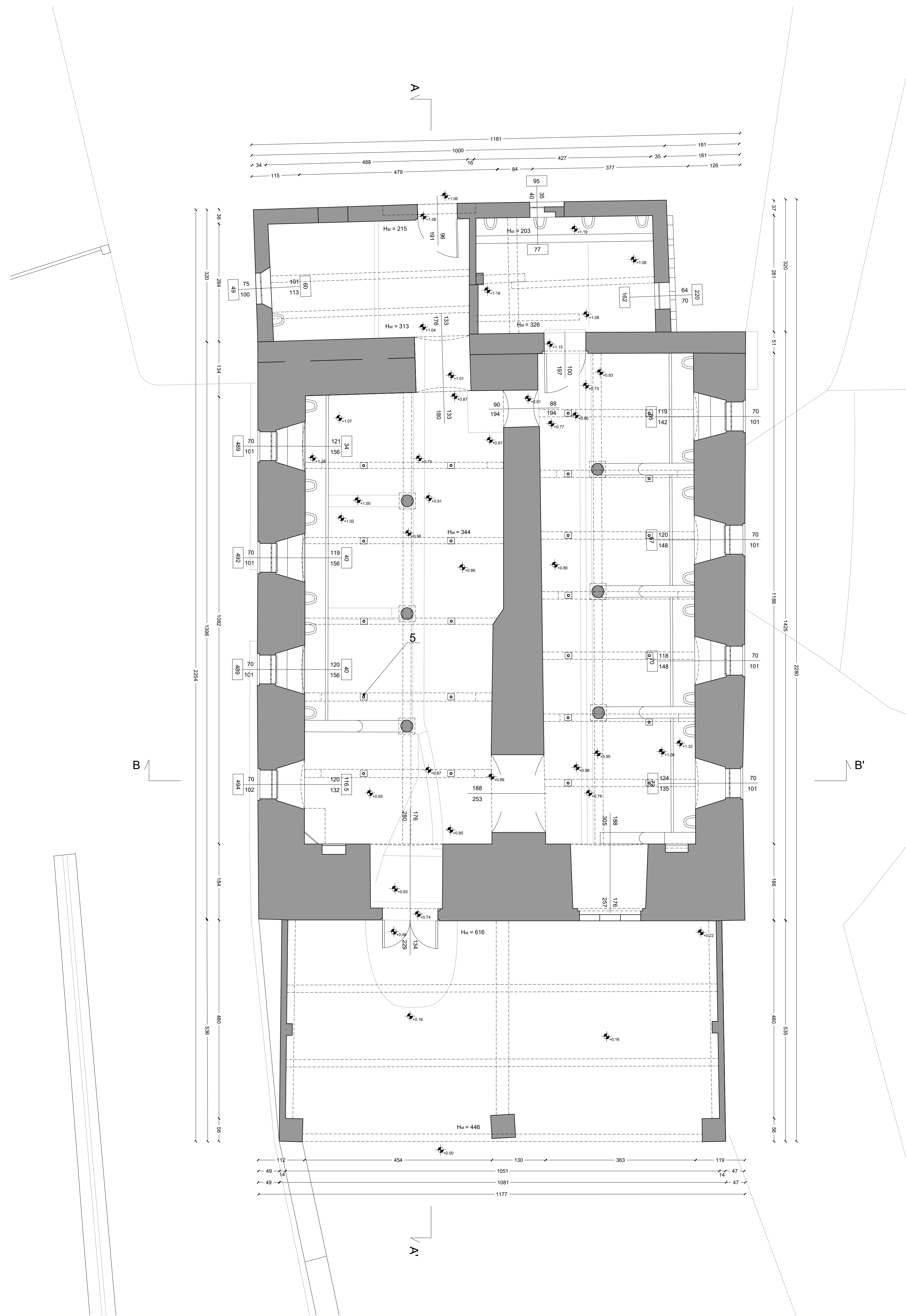
Stato di Progetto - Pianta Livello 0 - 1:50
