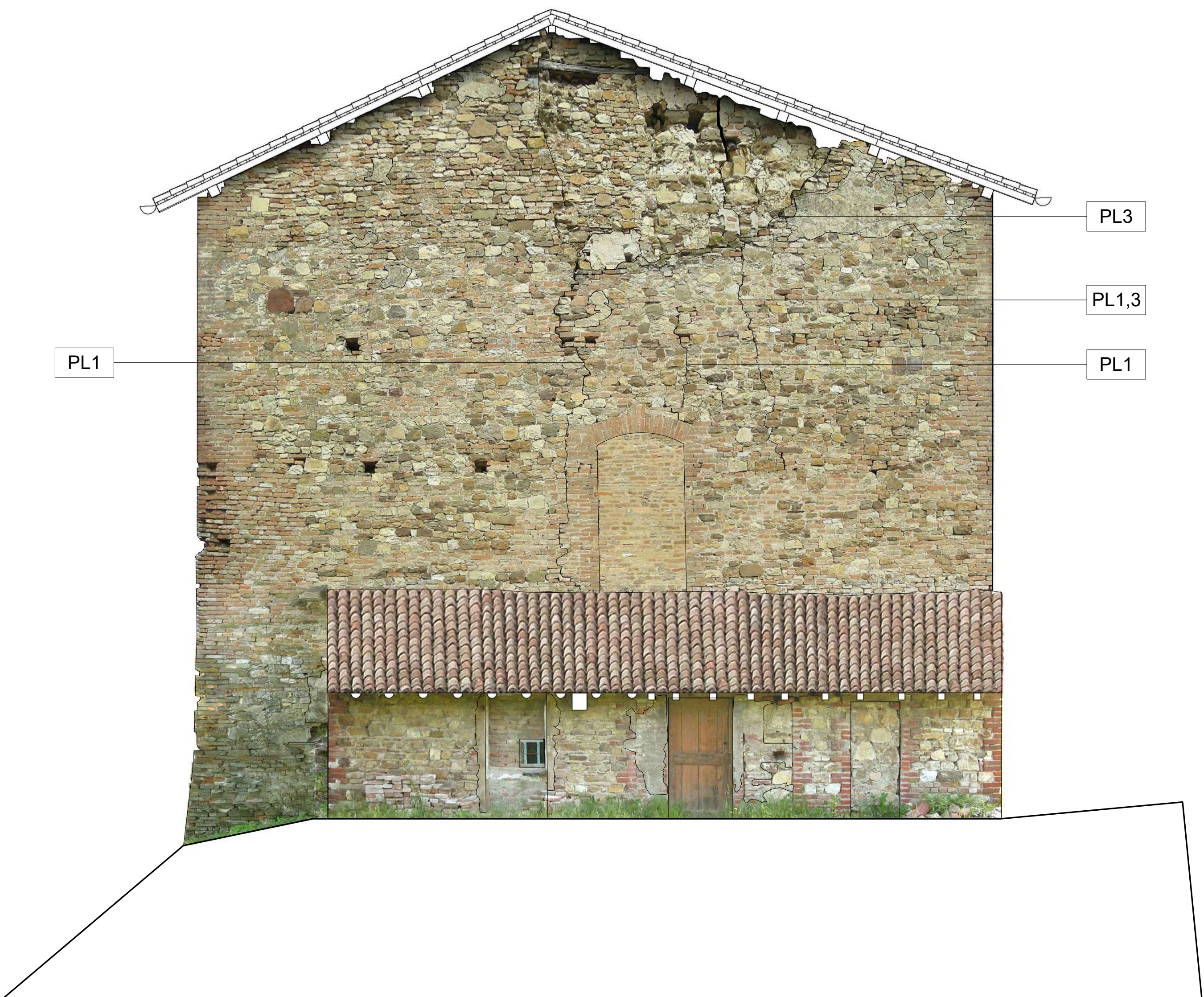
Prospetto Ovest - Degradi - Scala 1:50
