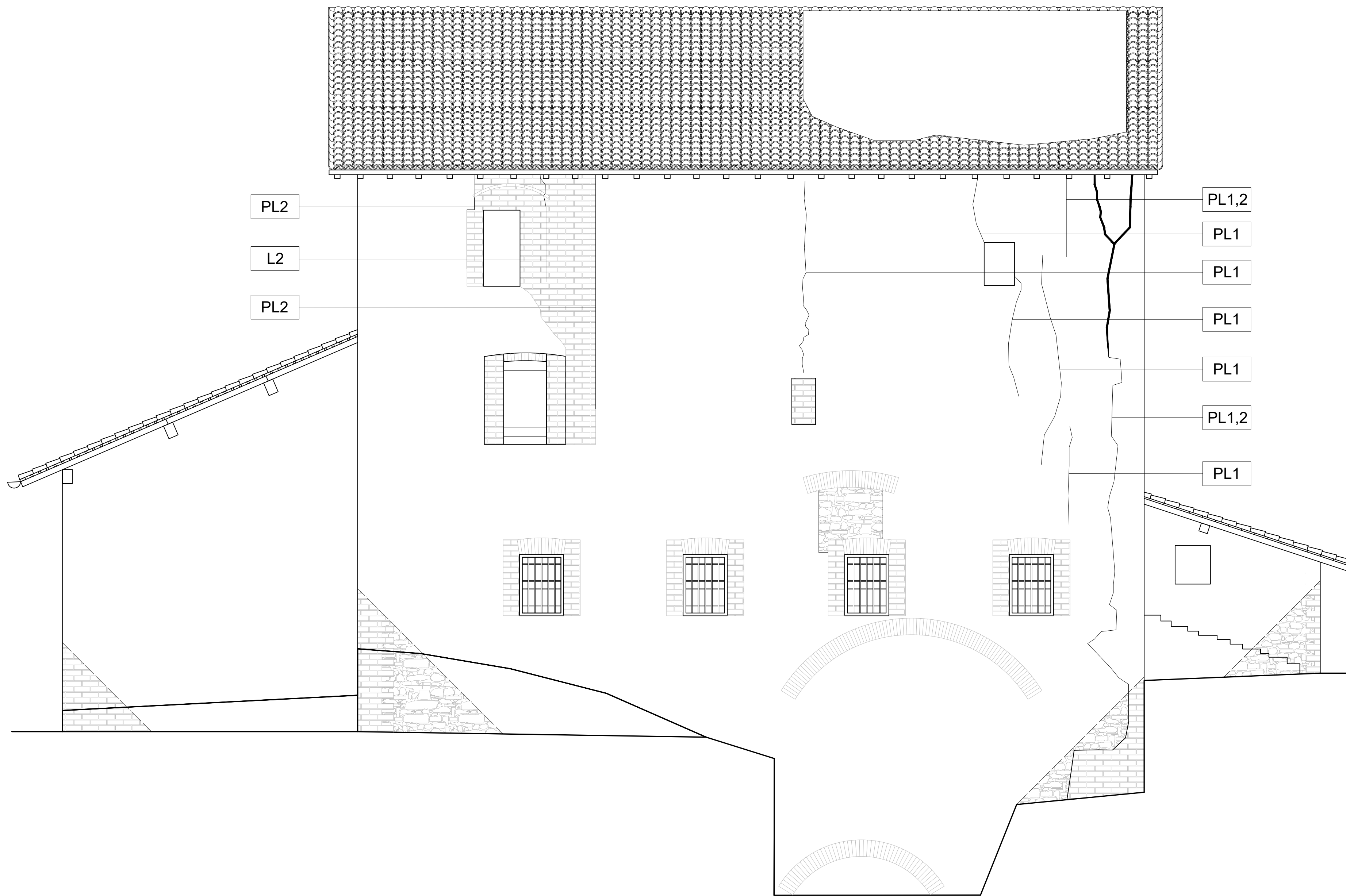
Prospetto Nord - Degradi - Scala 1:50
