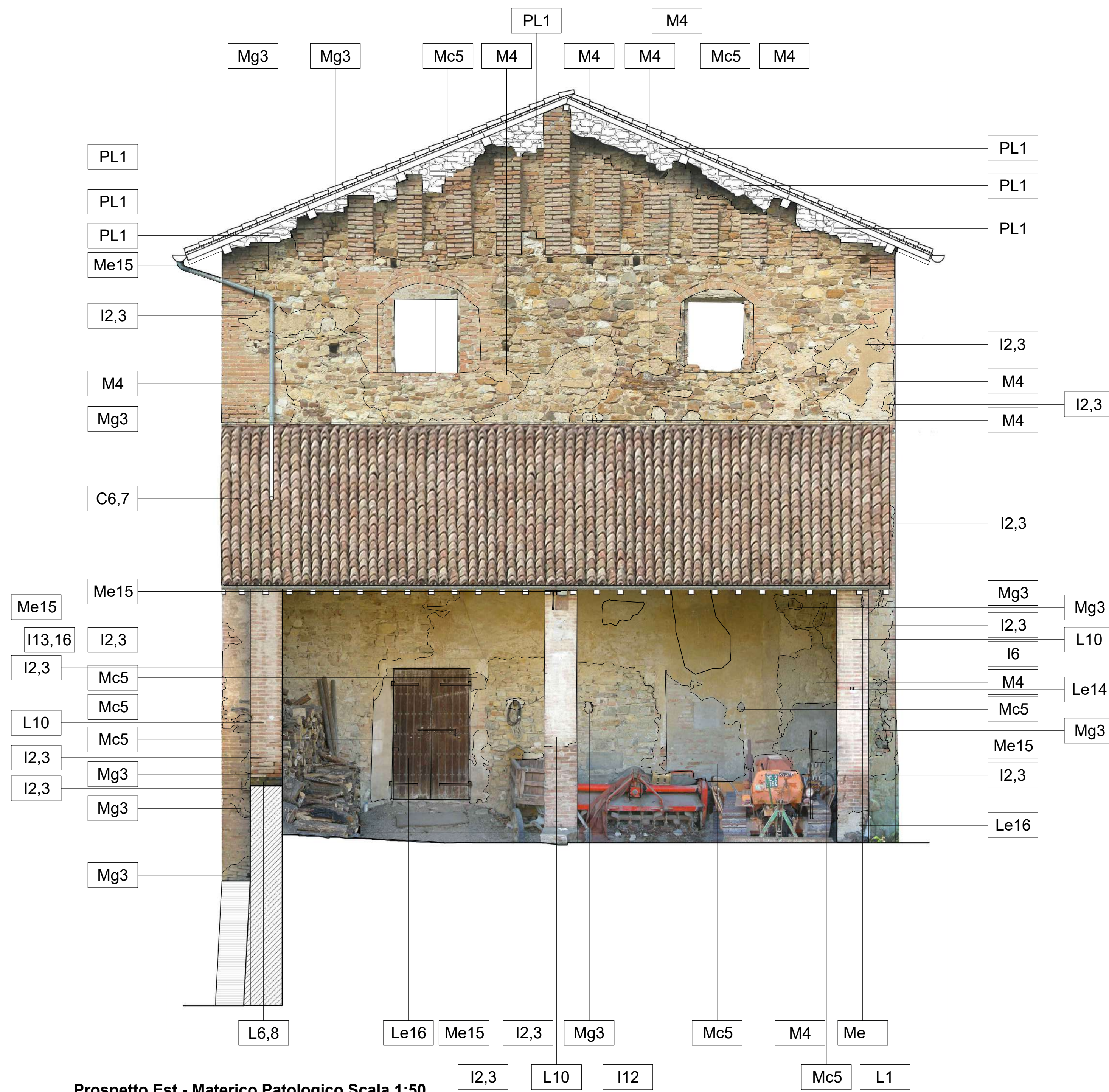
Prospetto Est - Materico Patologico Scala 1:50
