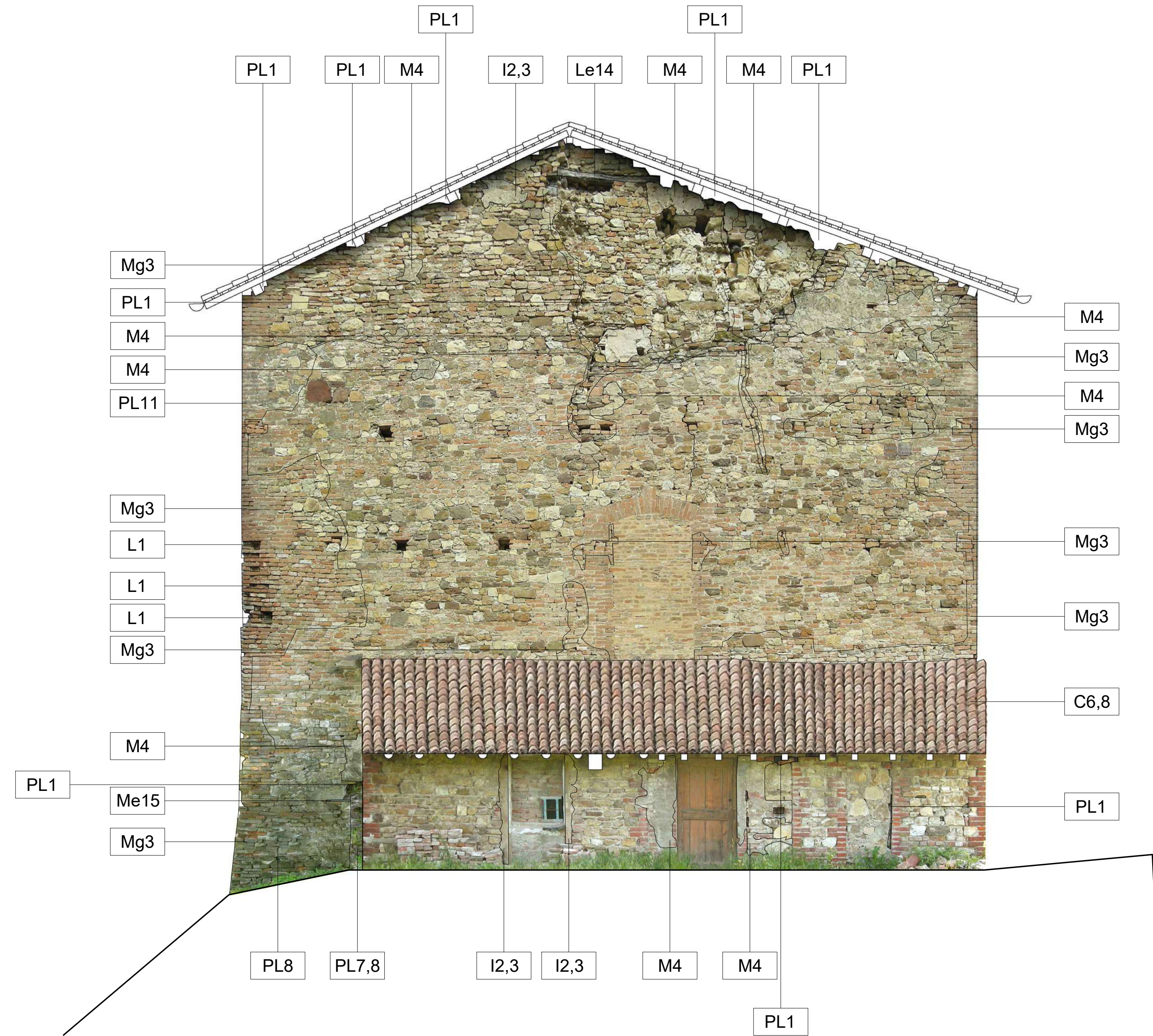
Prospetto Ovest - Materico Patologico - Scala 1:50
