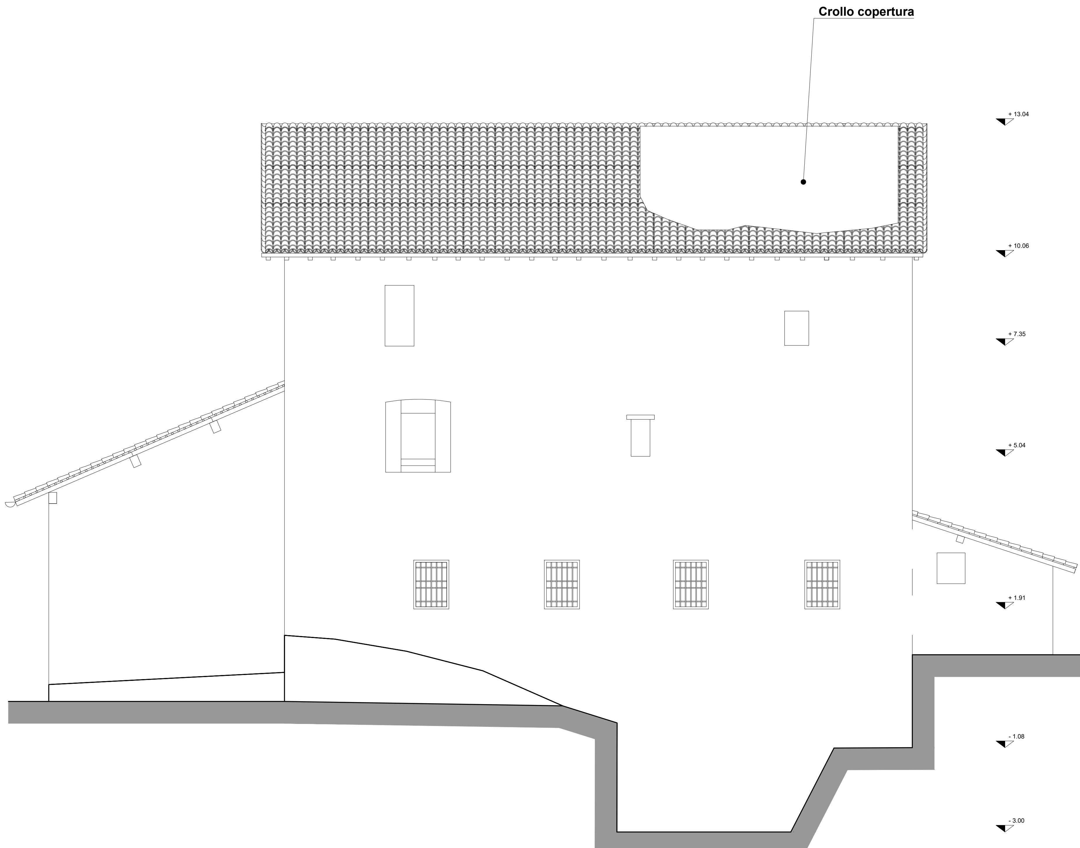
Prospetto Nord - Scala 1:50
