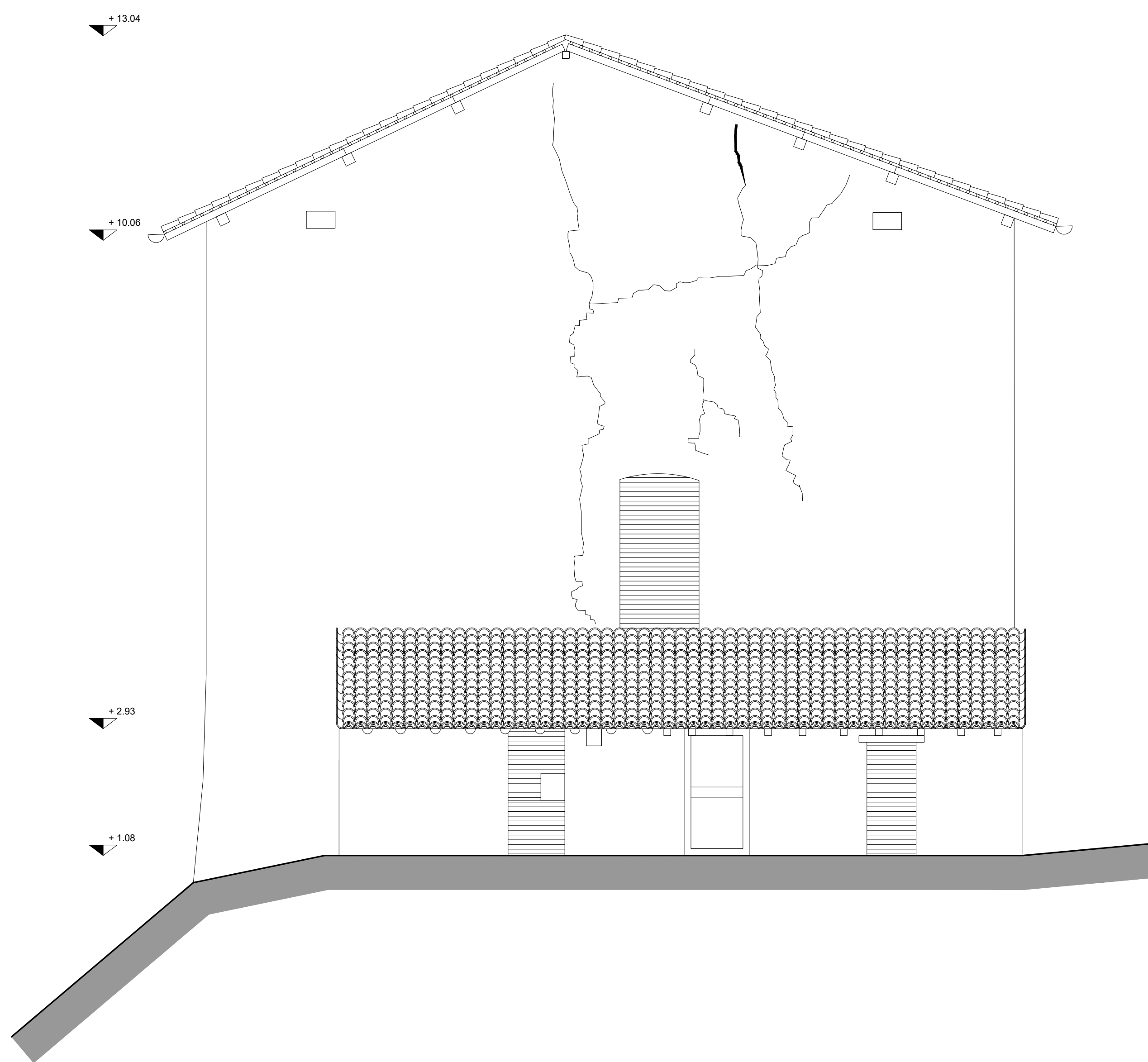
Prospetto Ovest - Scala 1:50
