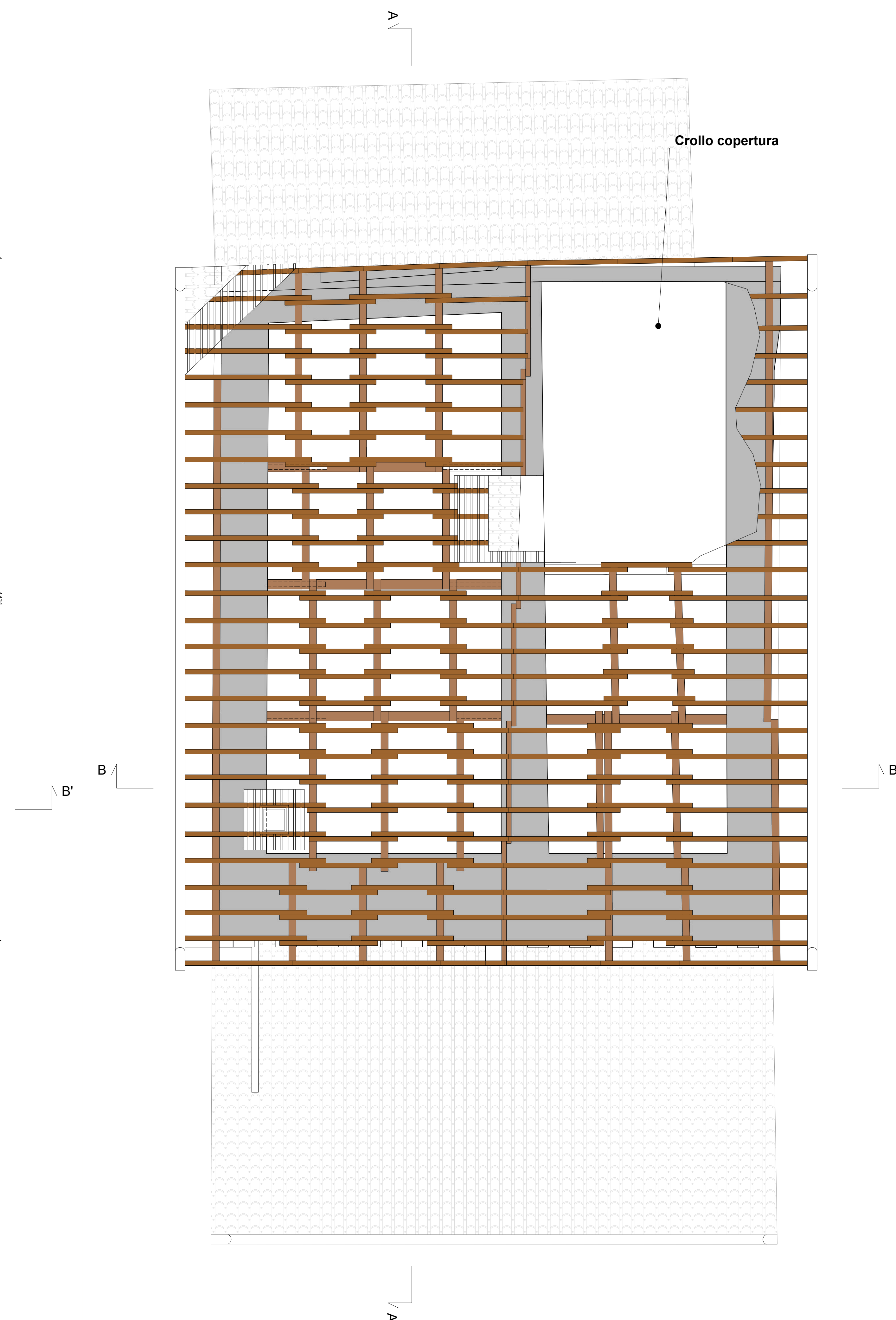
Stato di Fatto - Pianta Livello Copertura - 1:50
