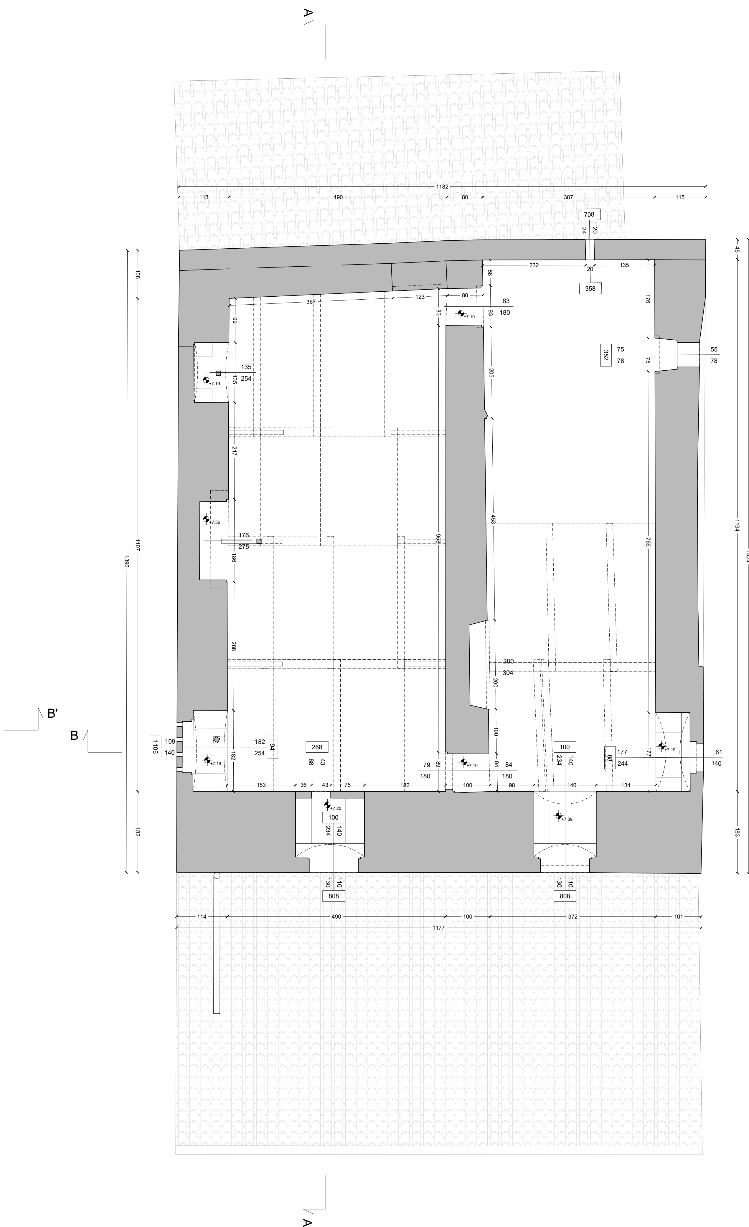
Stato di Fatto - Pianta Livello 2 - 1:50
