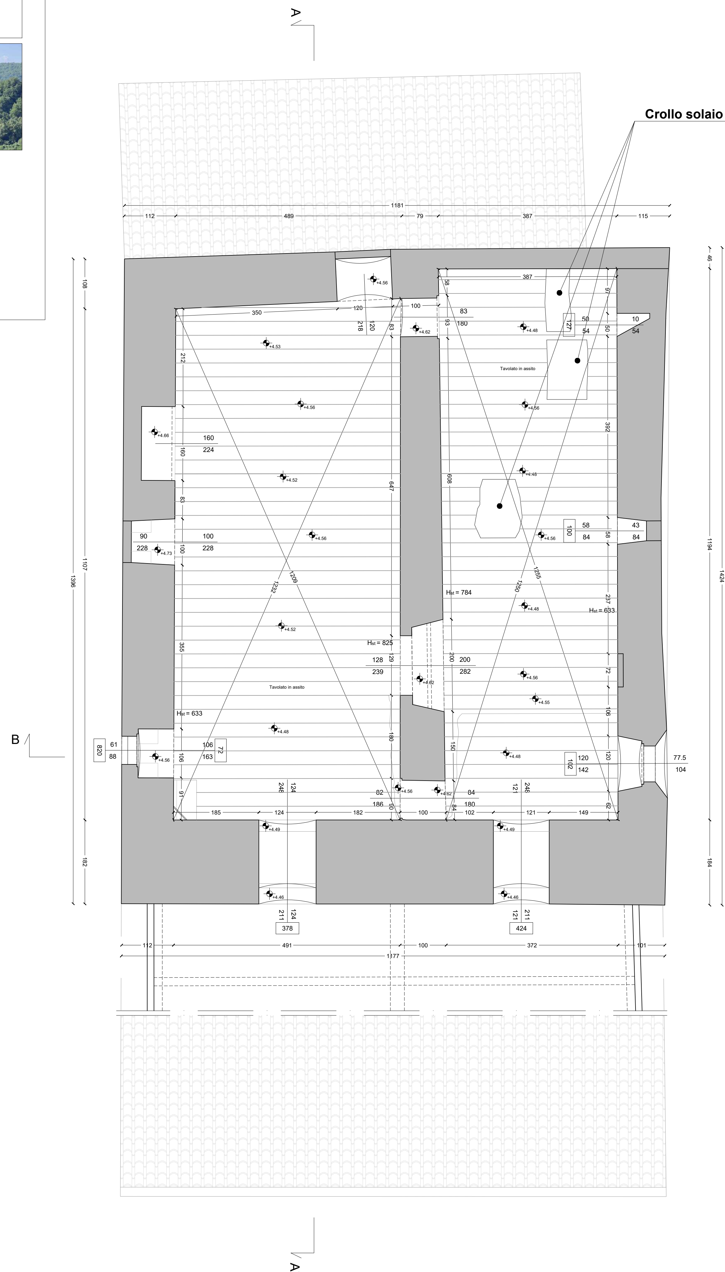
Stato di Fatto - Pianta Livello 1 - 1:50
