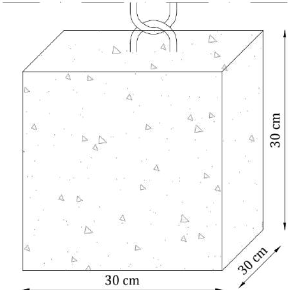
Particolare zavorra CLS armato
