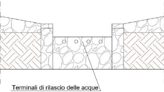
PROSPETTO NORD-EST DEL MANUFATTO DI REGOLAZIONE - fuori scala -
