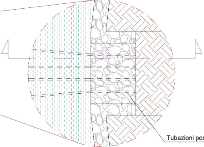
PARTICOLARE IN PIANTA DEL MANUFATTO DI REGOLAZIONE - fuori scala -
