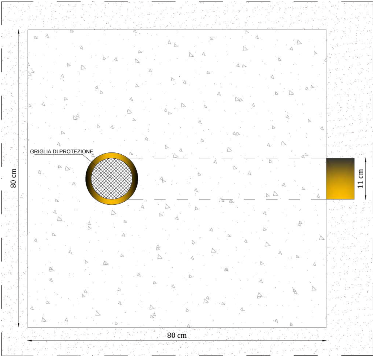
PARTICOLARE IN PIANTA DEL MANUFATTO DI PESCAGGIO IN CLS ARMATO
